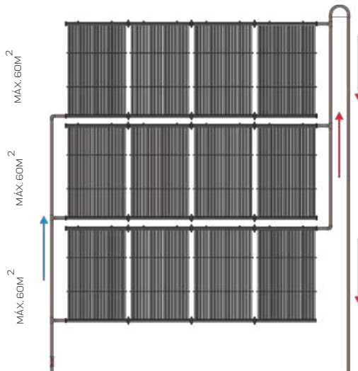
Exemplo de montagem de baterias em paralelo
