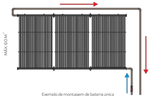
Exemplo de montagem de bateria única
